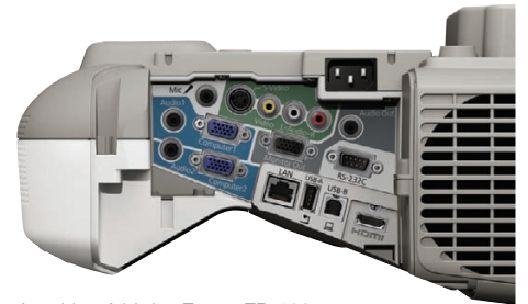
Anschlussfeld des Epson EB-480
